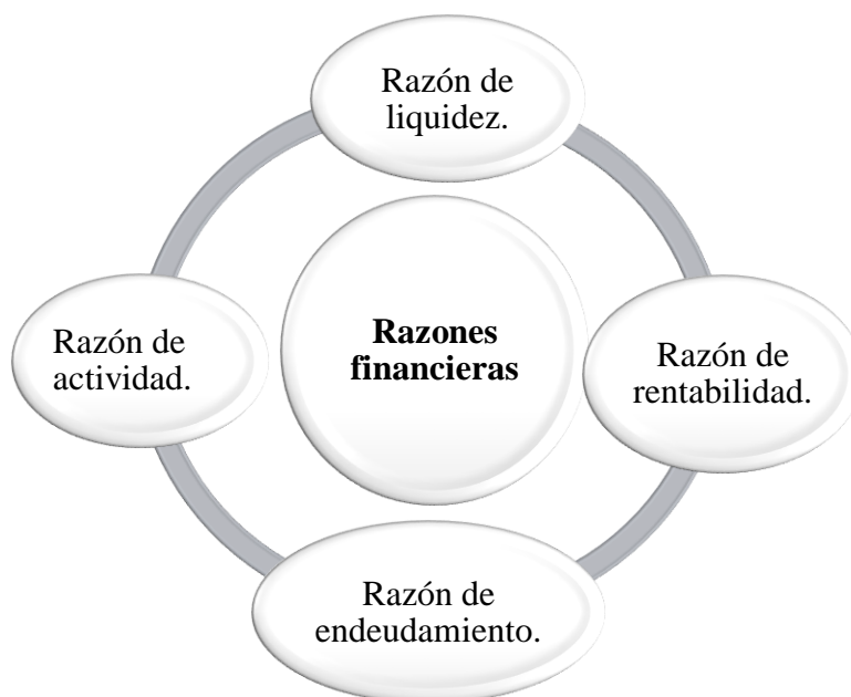
Figura 2: Razones financieras
